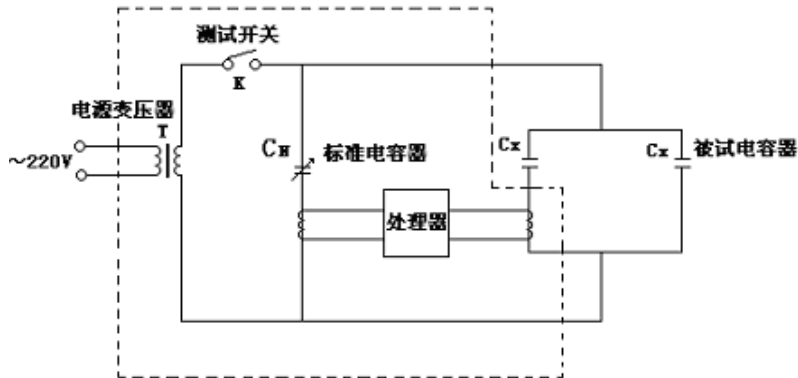
图1 电容电桥工作原理图
