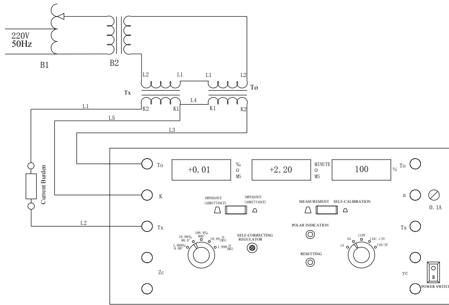
ii. 电压互感器误差试验接线原理图:
