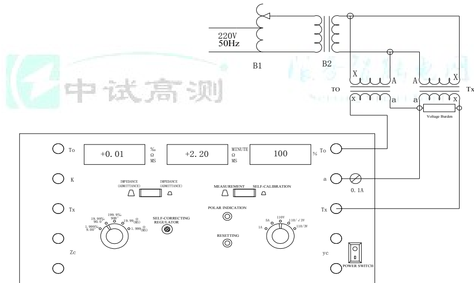
3. 电流互感器二次回路阻抗接线原理图:
