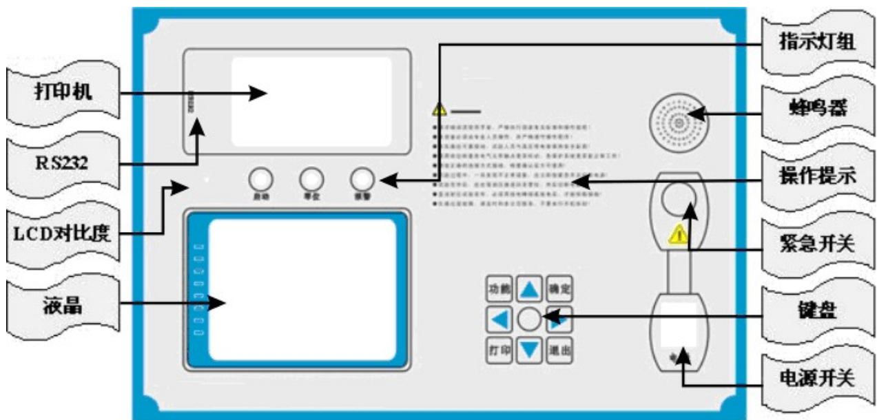
图 6 控制箱（台）面板结构图
