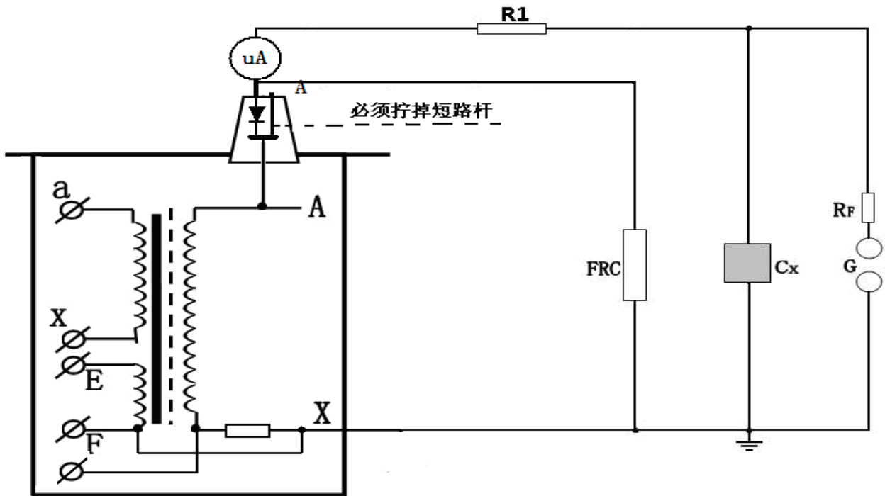
图中：R1—限流电阻 FRC—标准高压分压器 Rf—球隙保护电阻 G—保护球隙 Cx—被试品 uA—微安表
